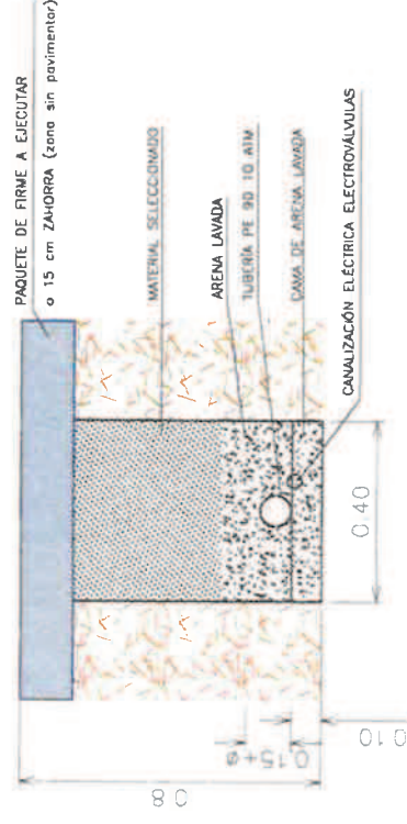
SECCIÓN TIPO DE ZANJA RIEGO
