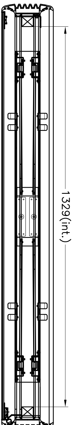
SECCION B-B
