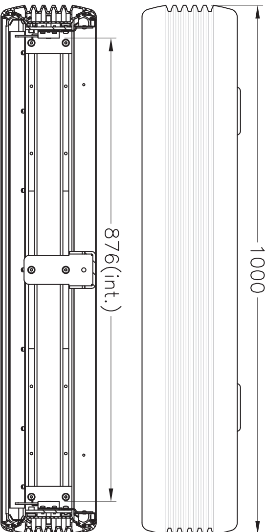
SECCIÓN B-B
