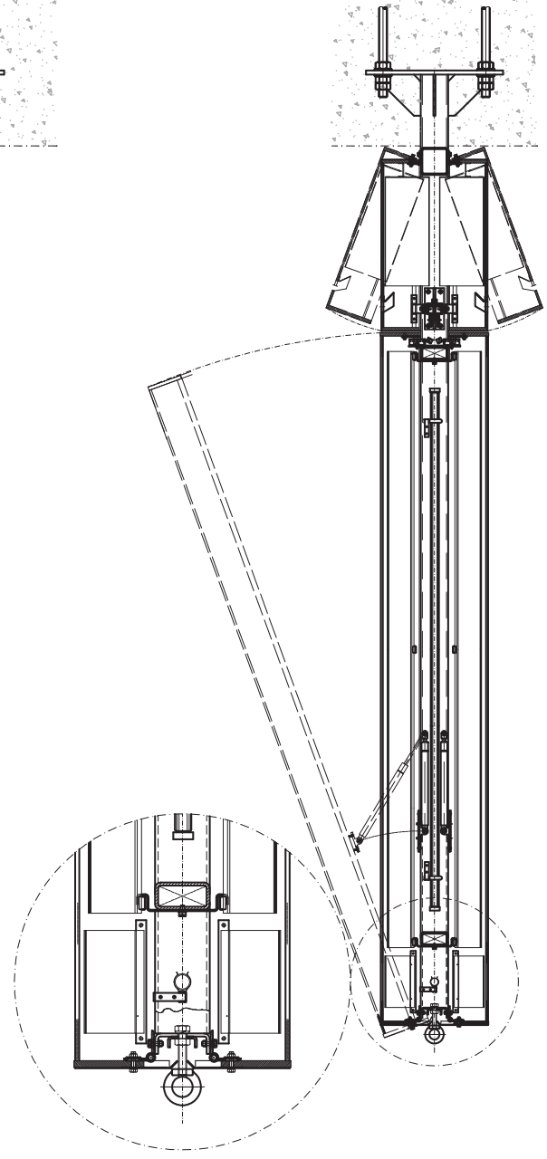
SECCION LATERAL
