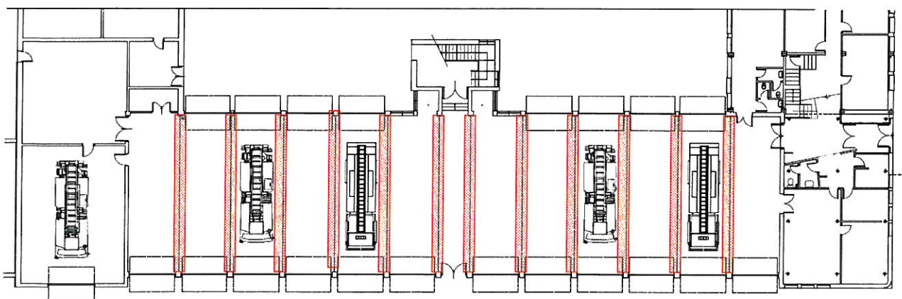
PLANTA BAJA
