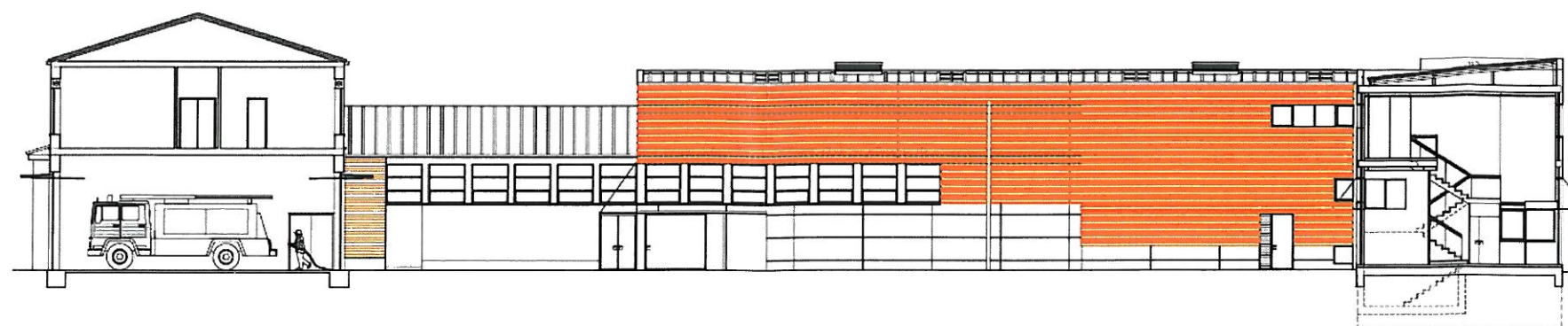
SECCIÓN N-S
