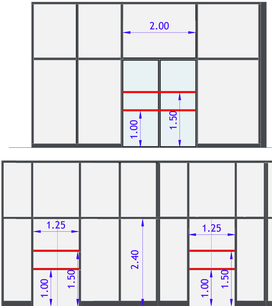
DETALLE PUERTA DEL MÓDULO DE ENTRADA EXTERIOR_E:1/50
