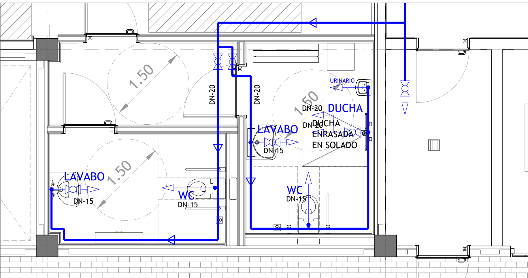
CUARTO DE BASURAS Y ASEOS PÚBLICOS ADAPTADOS EN PLANTA BAJA_E 1/40
