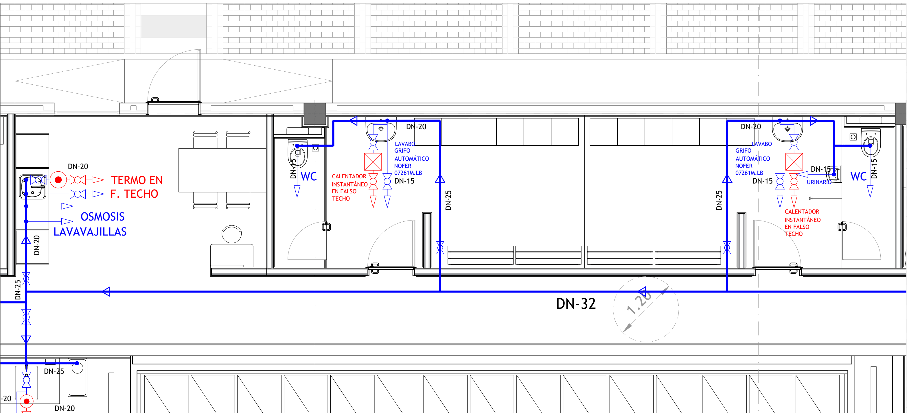
VESTUARIOS DE DEPENDENCIAS Y SALA DE DESCANSO EN PLANTA BAJA_E 1/40
