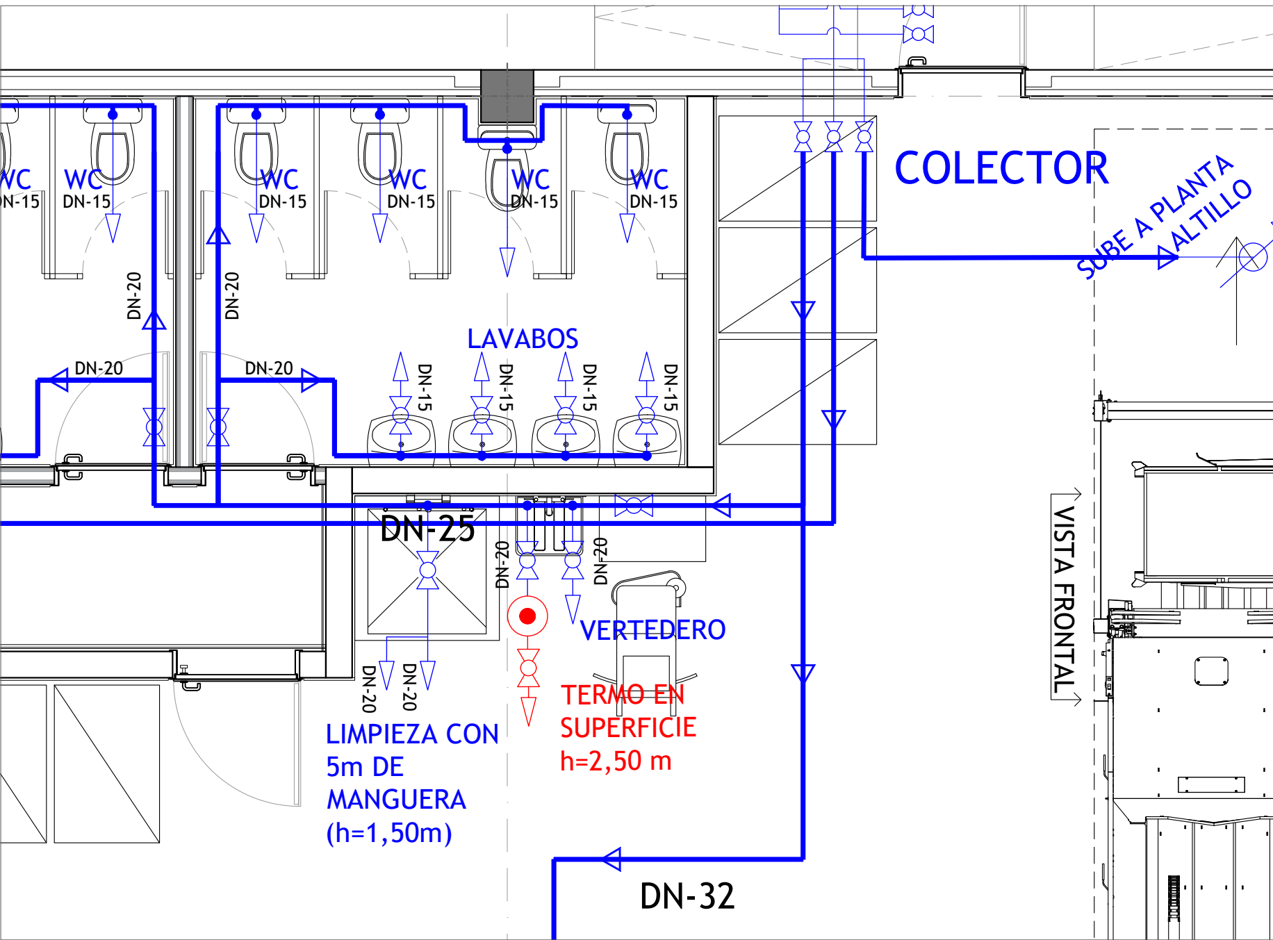
VERTEDERO Y ZONA DE LIMPIEZA DE ALMACÉN_E 1/40
