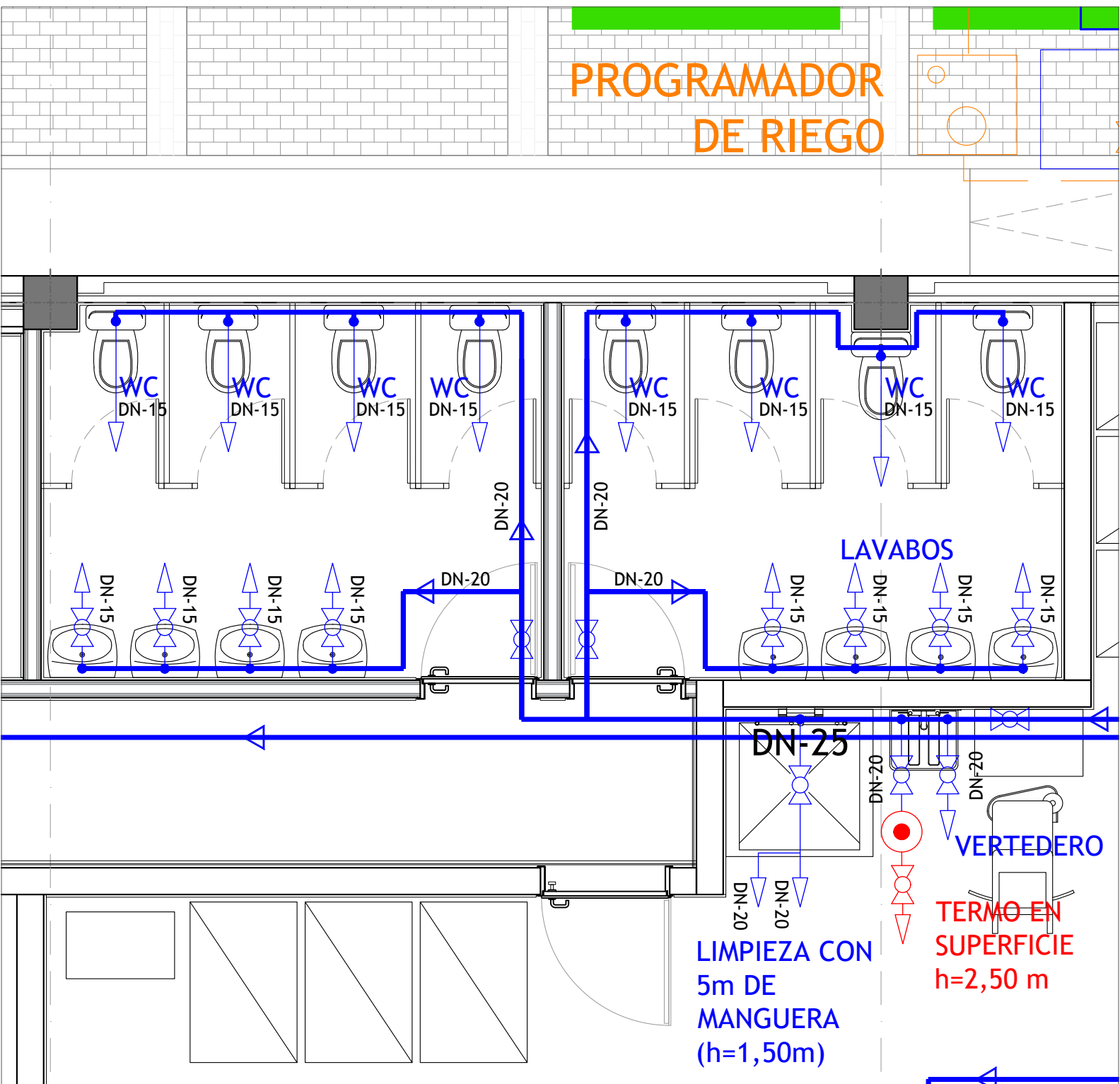
ASEOS DOTACIONALES EN PLANTA BAJA_E 1/40
