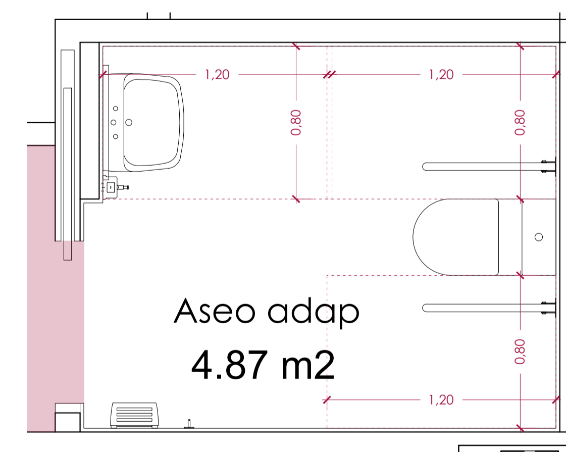
ASEO ADAPTADO DE USO PÚBLICO
