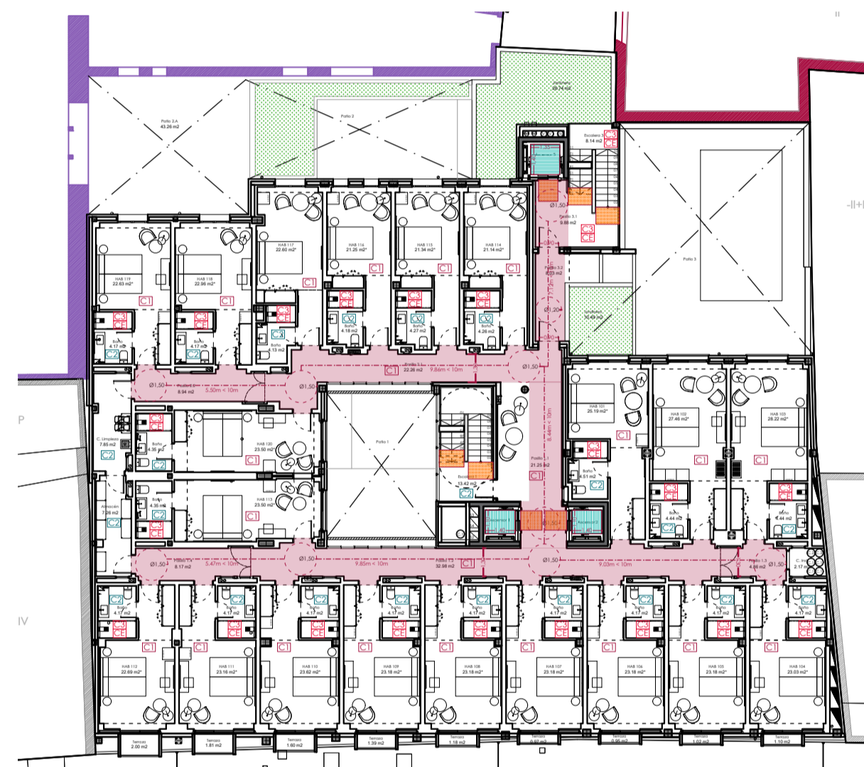
PLANTA PRIMERA
