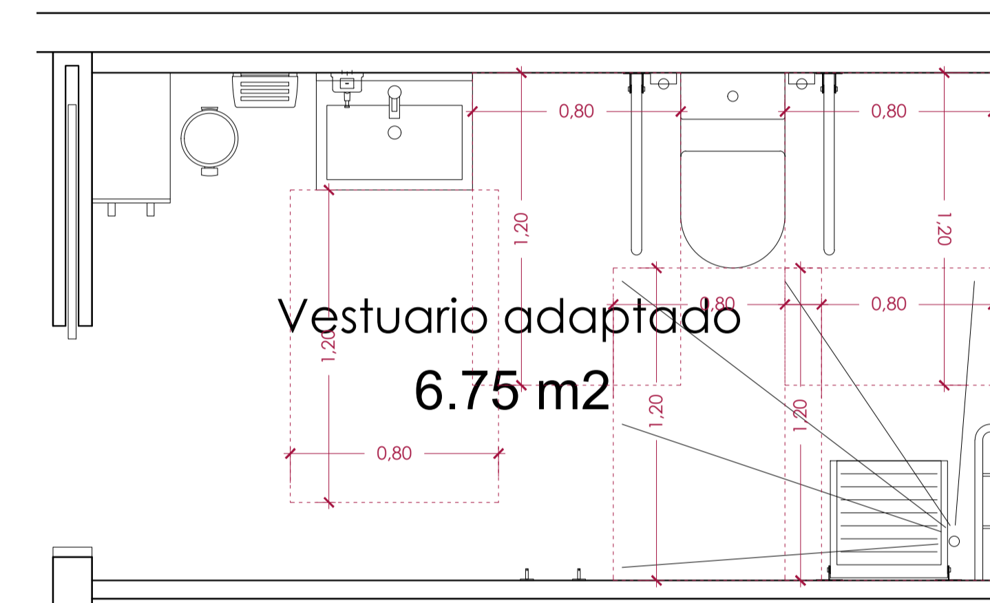
VESTUARIO ADAPTADO DE USO PRIVADO DE TRABAJADORES
