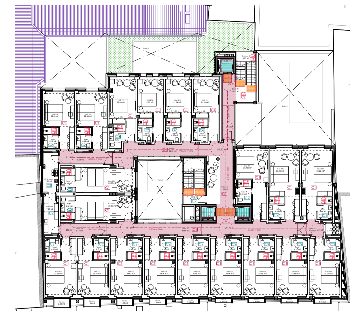
PLANTA SEGUNDA
