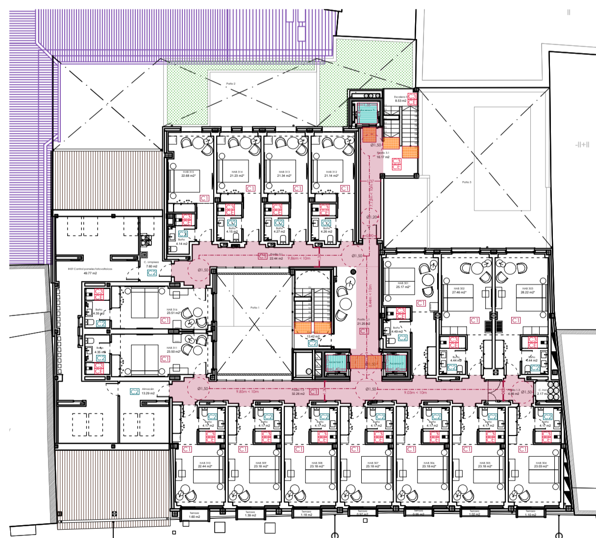
PLANTA TERCERA
