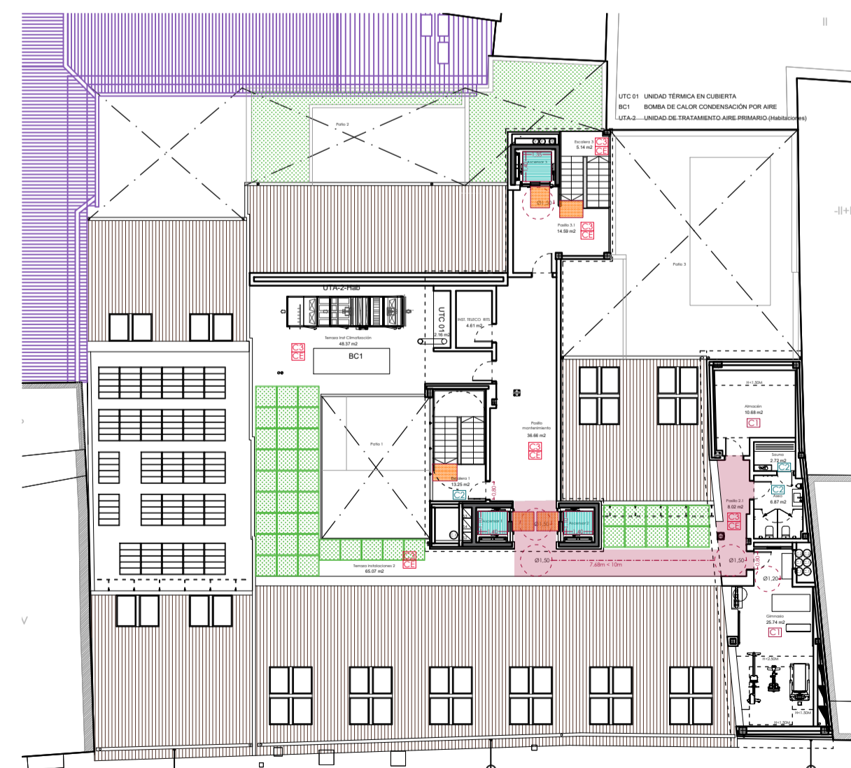
PLANTA CUBIERTA
