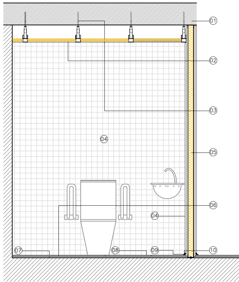
DETALLE ASEO MINUSVALIDOS
