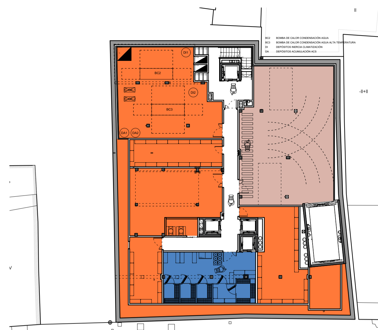
PLANTA SÓTANO -2
