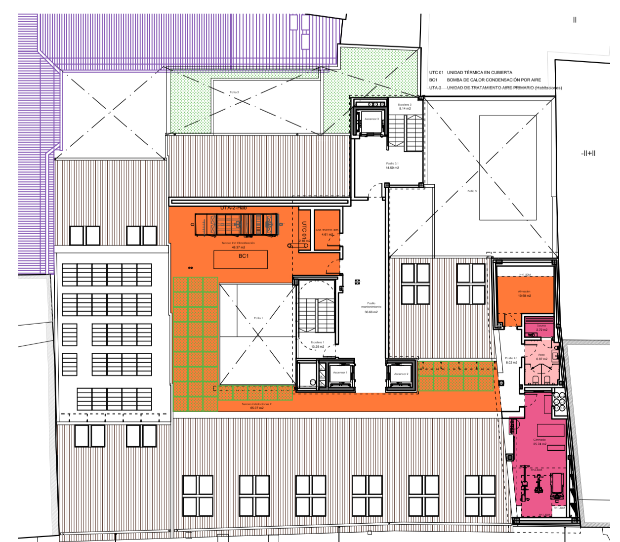
PLANTA CUBIERTA
