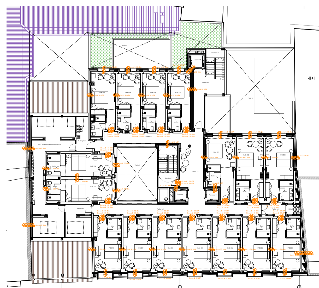
PLANTA TERCERA
