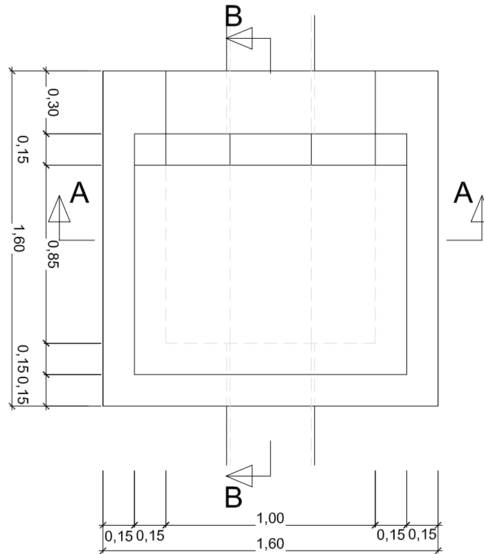
PLANTA ESCALA 1:25 ( cotas en cm.)
