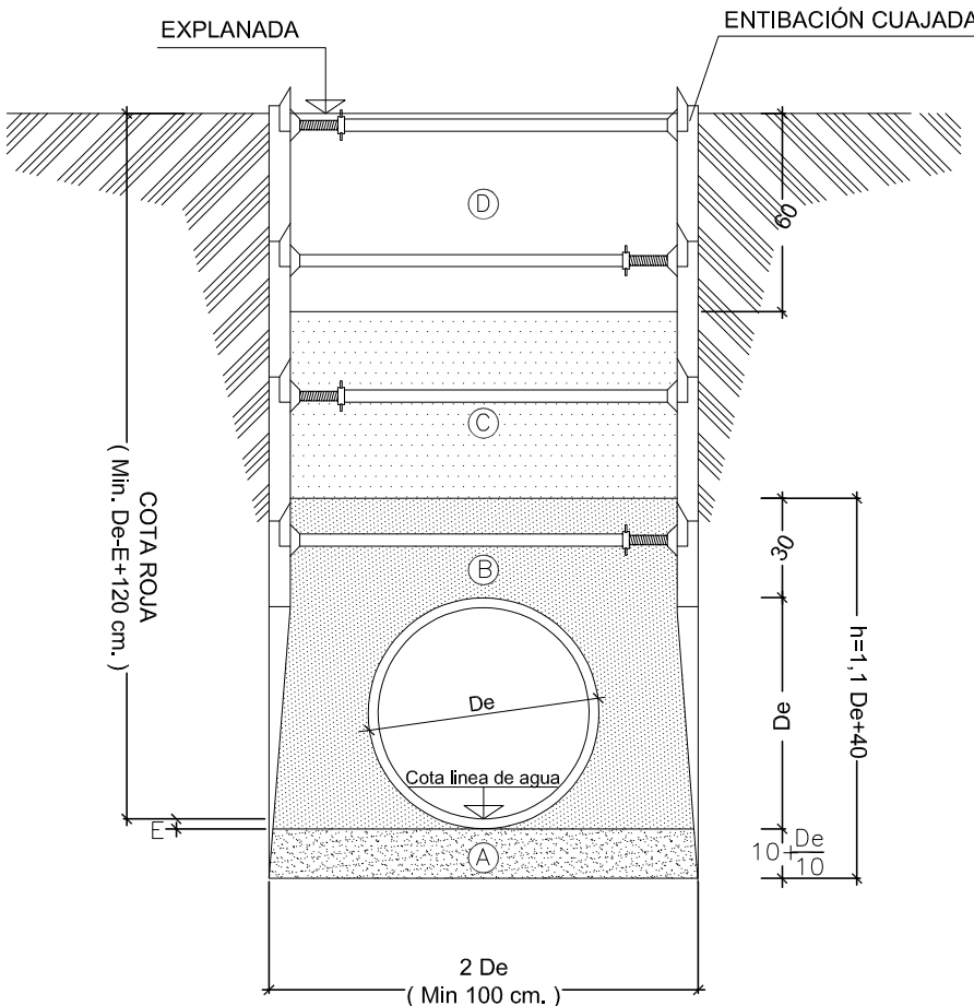
SECCION TIPO DE ZANJA ENTIBADA ( CAMA GRANULAR )
