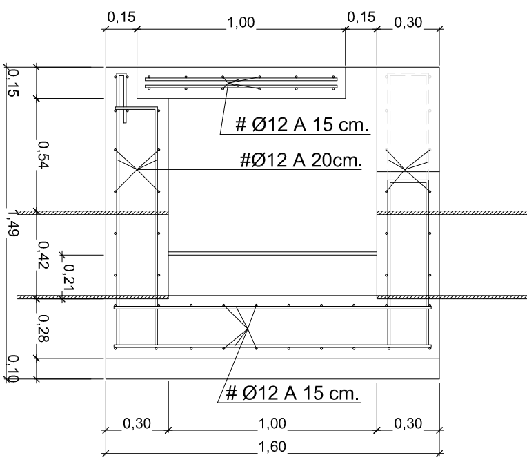
SECCION B-B ESCALA 1:25 ( cotas en cm.)
