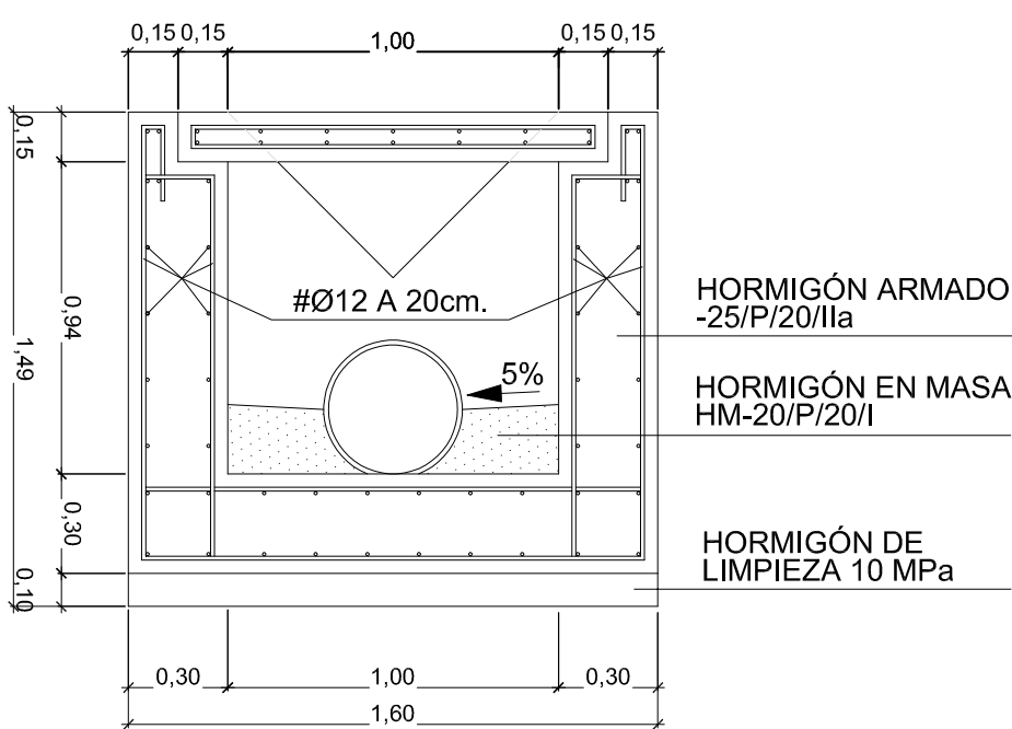
SECCION A-A ESCALA 1:25 ( cotas en cm.)
